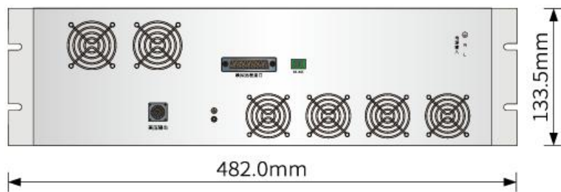
后视图
