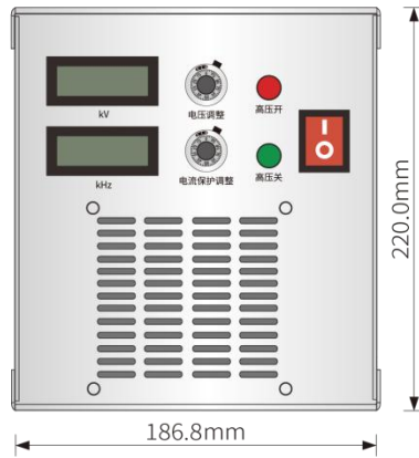
主视图
