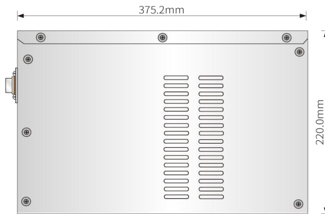
侧视图
