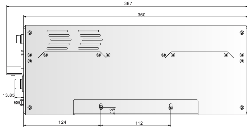
侧视图
