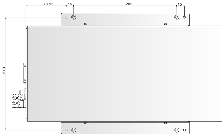
俯视图
