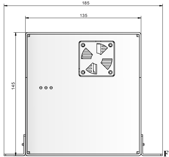
后视图
