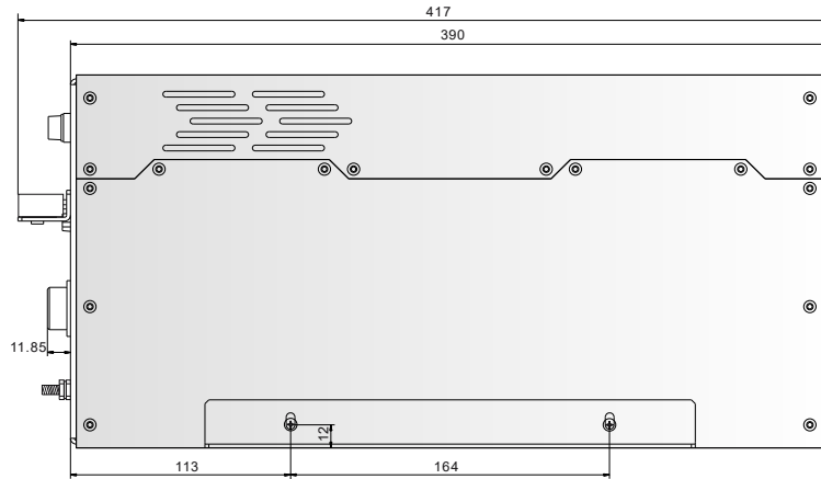
侧视图
