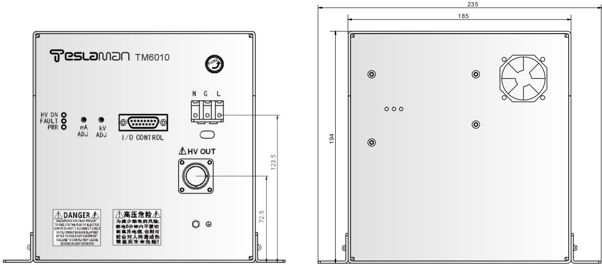
前视图
