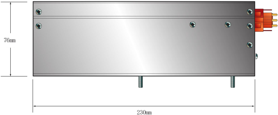
侧视图
