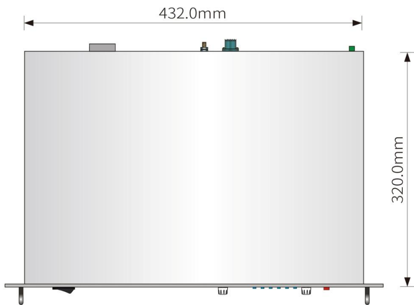
俯视图
