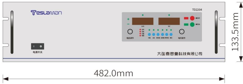
主视图
